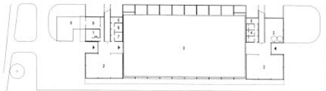
NOUVEAU BATIMENT REZ INFÉRIEUR 1/300
