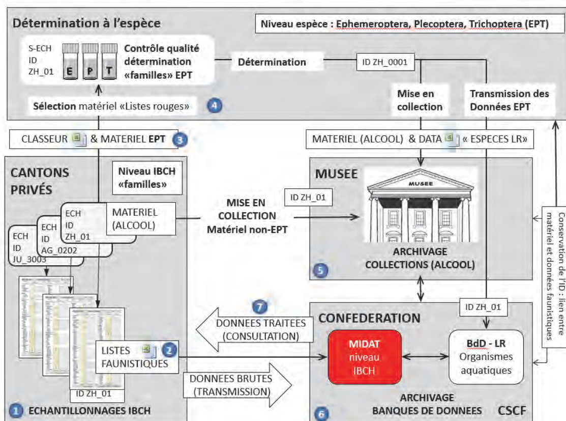
Figure 7 : Schéma présentant les étapes de valorisation et archivage des échantillonnages IBCH:
