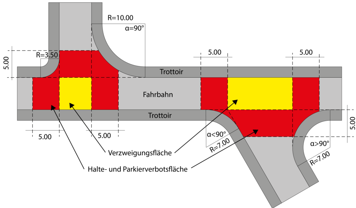
Abbildung 1: Halte- und Parkierverbotflächen bei Verzweigungen
