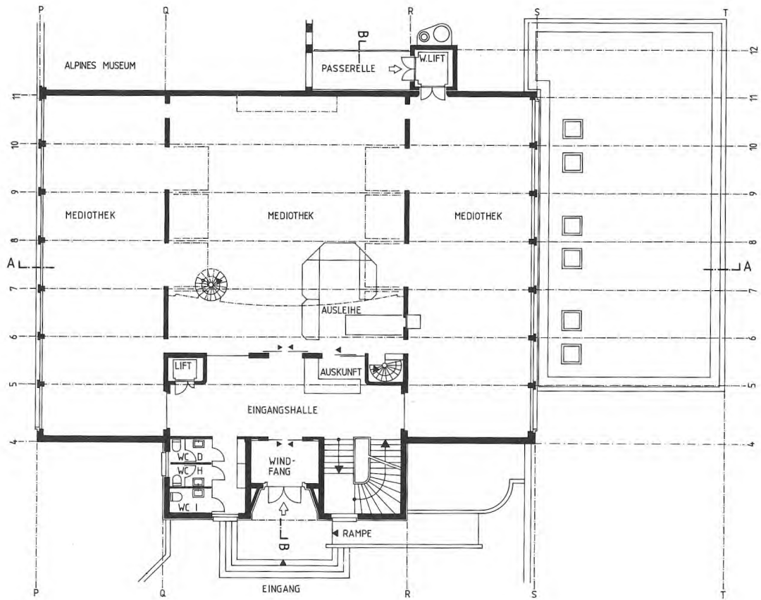
ERDGESCHOSS
