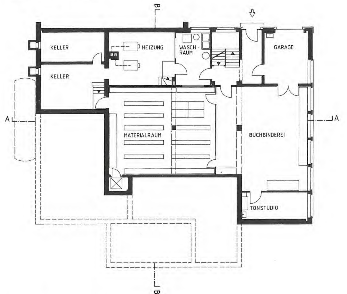
2. UNTERGESCHOSS
