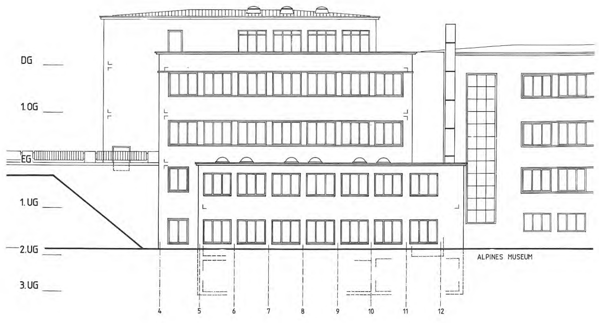
NORDFASSADE
