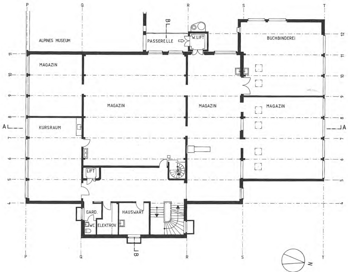
1. UNTERGESCHOSS
