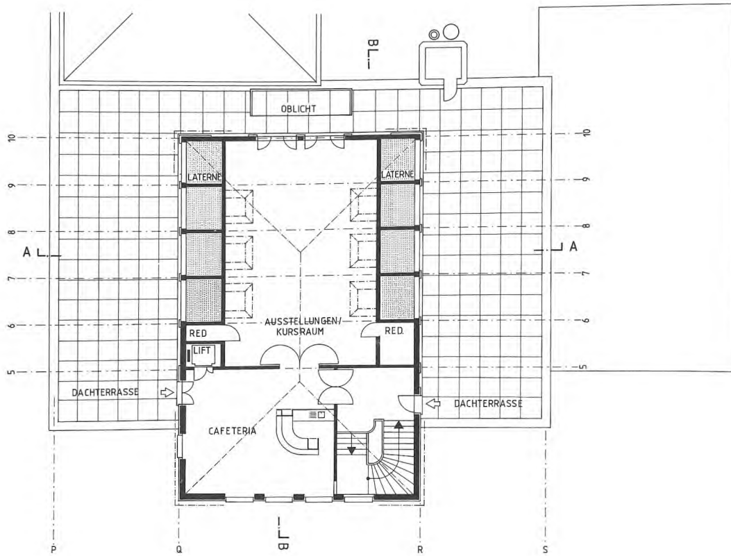
DACHGESCHOSS
