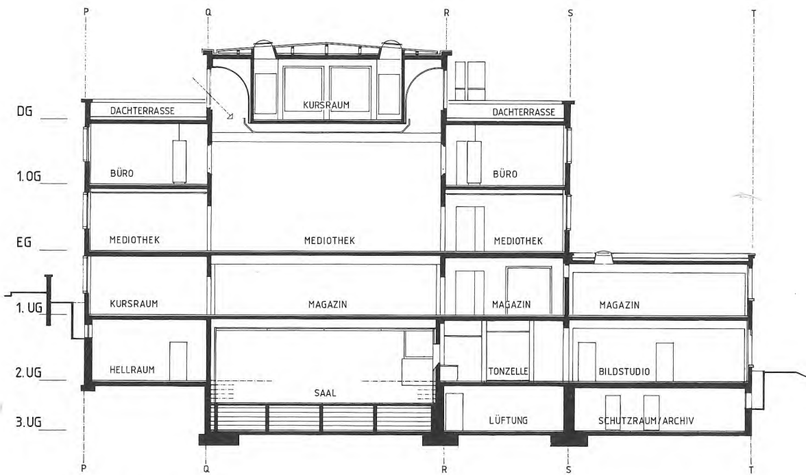
QUERSCHNITT A_A
