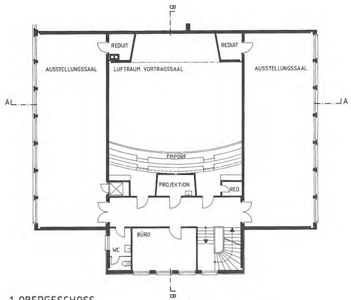
1. OBERGESCHOSS
