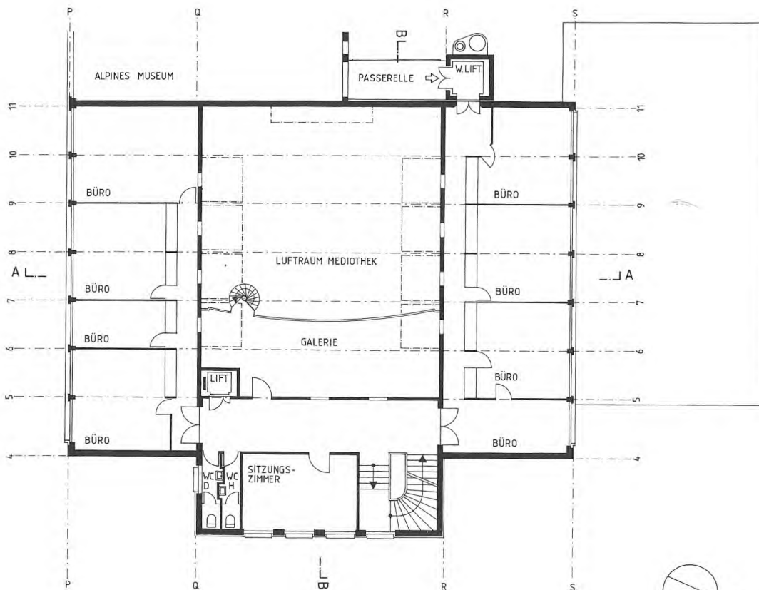
1.OBERGESCHOSS
