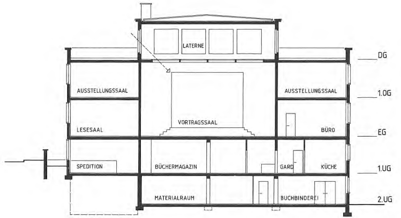
QUERSCHNITT A-A
