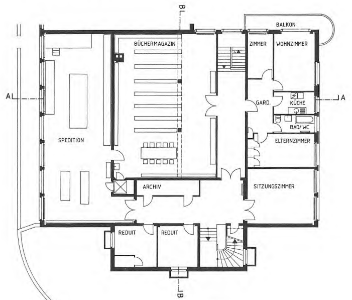
1. UNTERGESCHOSS
