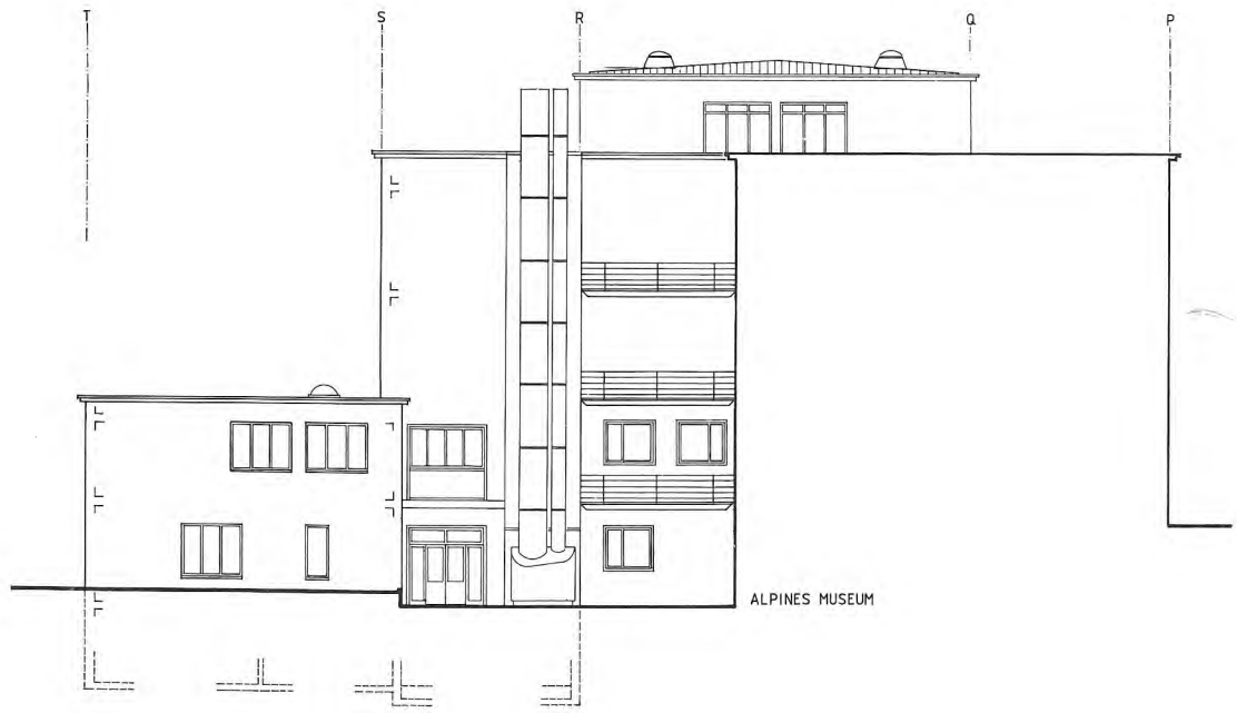
WESTFASSADE
