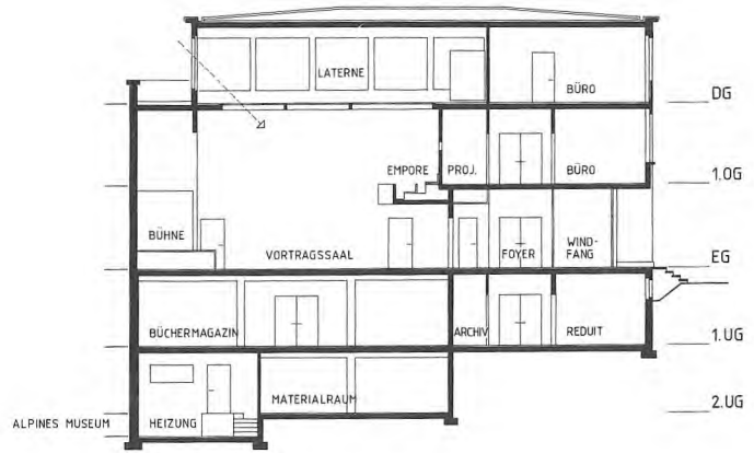
LÄNGSSCHNITT B_B
