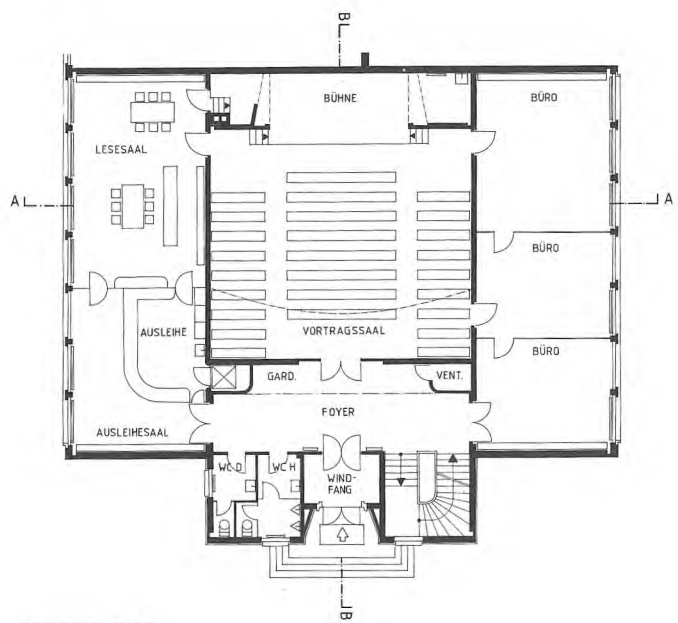
ERDGESCHOSS
