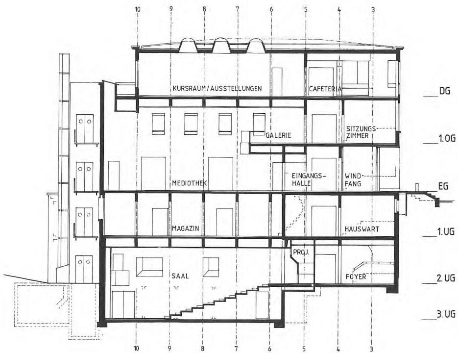
LÄNGSSCHNITT B_B
