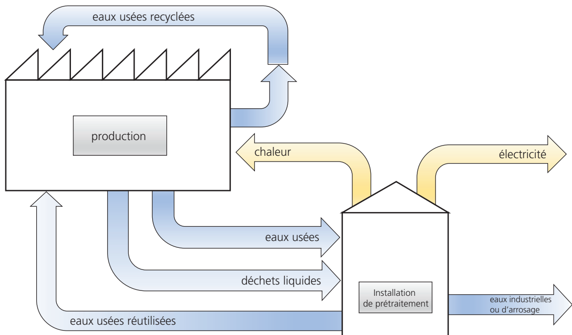
Figure 4 : Exemple d'une gestion globale des ressources. En bleu : circuit d'eau, en jaune : flux d'énergie.
