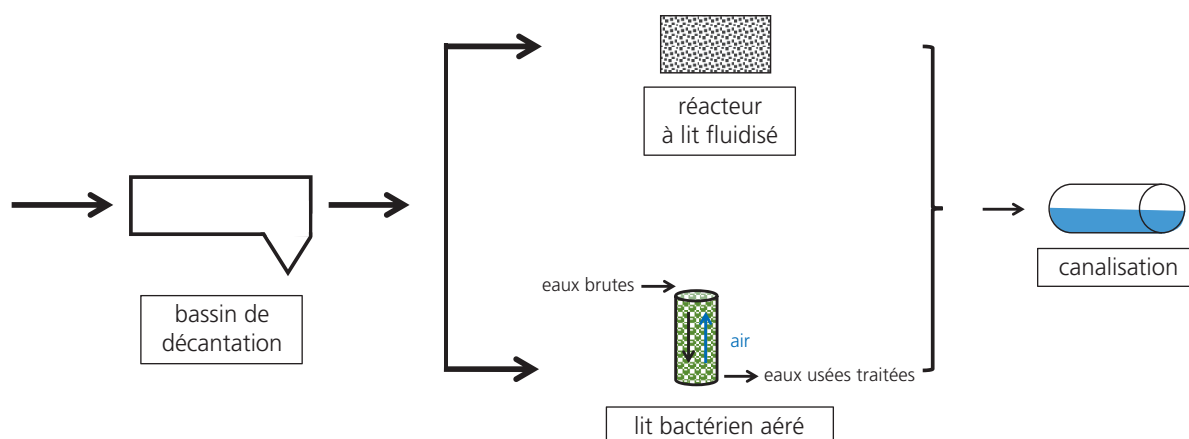
Figure 5 : graphique: tbfpartner Aperçu des procédés pour des eaux usées moyennement chargées qui sont déversées dans les égouts après un prétraitement.
