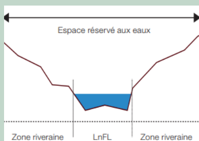
Figures 3 et 4 : Représentation schématisée d'un cours d'eau (à gauche) et d'une étendue d'eau (à droite), avec leurs zones riveraines et espace réservé aux eaux. LnFL : = Largeur naturelle du fond du lit
